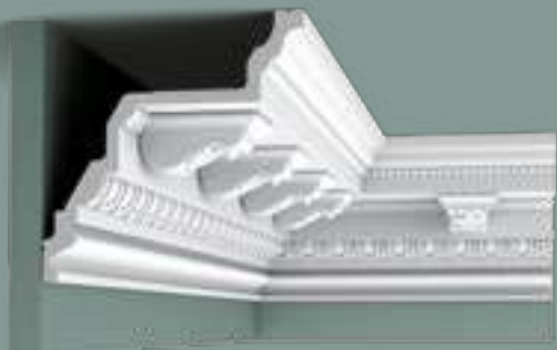
1 C307 + C307A 2 C307A: 7,5 x 4 x 9,4 Duropolymer® 19,5 9,4 4 5,6 ∇ = 26,9
