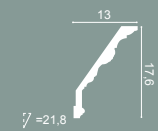
C219 200 x 17,6 x 13 cm Purotouch®
