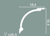
C338B BA'ROCK 200 x 18,4 x 18,4 cm Purotouch®
